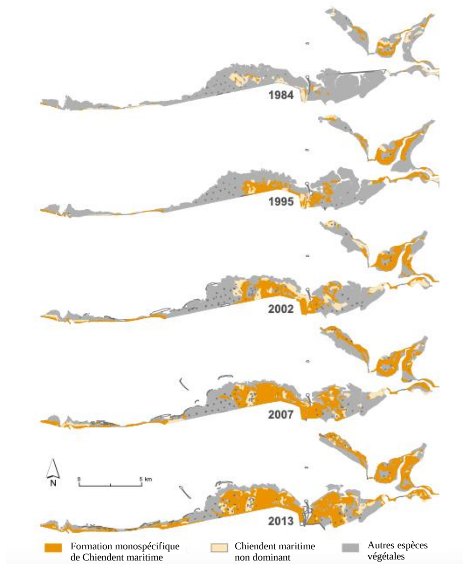
Figure 10 : Évolution des superficies de Chiendent maritime entre 1984 et 2013. Source = Valéry et Radureau, 2014
